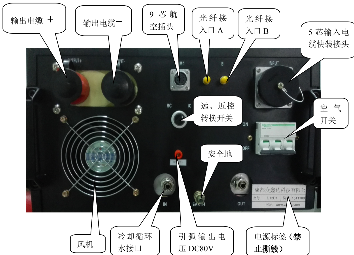
电源后面板示意图 (图二)
