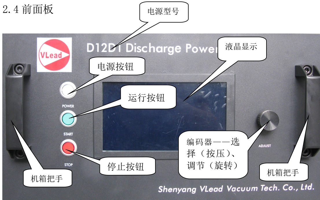
电源前面板示意图（图一）
